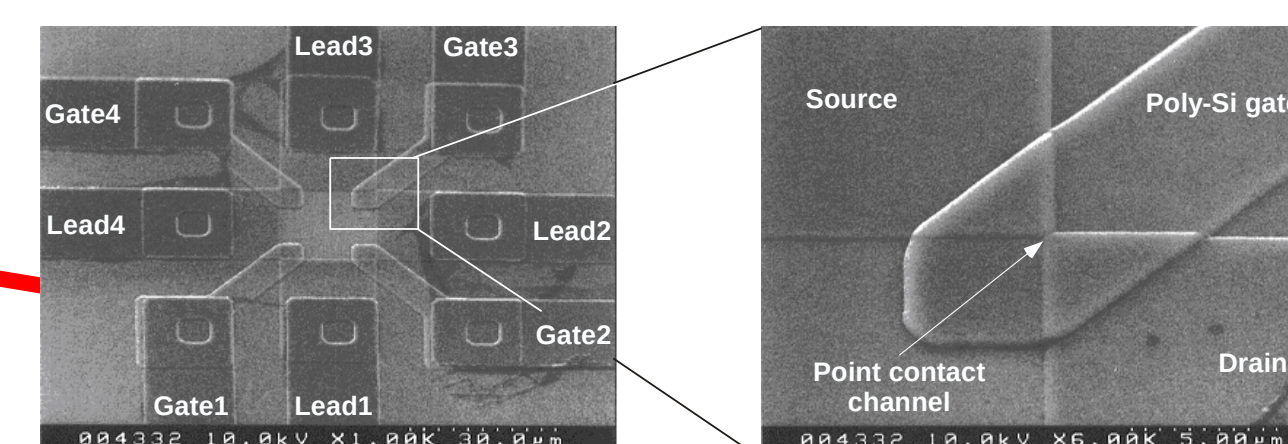
Fig. 7. Beyond CMOSの一種である室温動作の単電子トランジスタの集積化とCMOSとの融合に世界で初めて成功。量子コンピュータ向けの量子ビットに応用。
