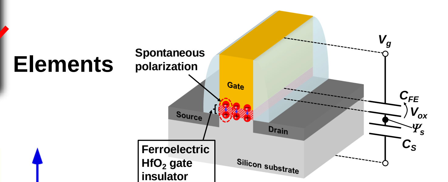
Fig. 6. 物理限界を突破して急峻なサブスレショルド特性を実現する負性容量トランジスタ技術。
